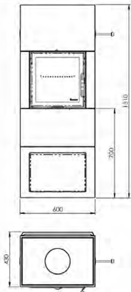
Salzburg S - záklop žárobeton/se zásobníkem na dřevo
